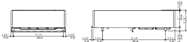
Oldalnézet
